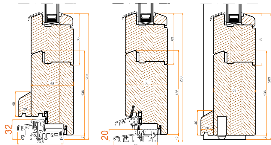
Próg aluminiowy GUTMANN 74/32 TI
