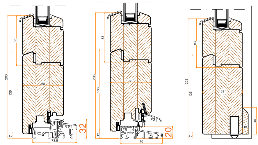
Próg aluminiowy GUTMANN 74/32 TI
