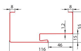
Ościeżnica stalowa z uszczelką do drzwi stalowych zewnętrznych 72 LUX FD-25/21B-72
