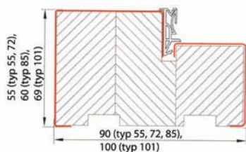
Ciepła ościeżnica stalowo-drewniana z uszczelką do drzwi stalowych zewnętrznych 55, 55 LUX, 72 LUX, 72 LUX TERMO, 85 LUX TERMO PLUS, 101 LUX TERMO PLUS
