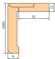
Opaska kątovej 60/80 mm z klipsem MDF za dopłatą
