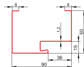
Ościeżnica stalowa z uszczelką do drzwi stalowych zewnętrznych 55, 55 LUX FD-25/21B-55
