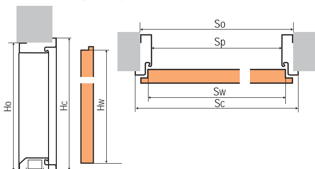
Rys. nr 1 Osadzenie ościeżnicy narożnej na mur
