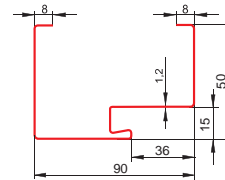
Ościeznica stalowa z uszczelką FD-25/21B
