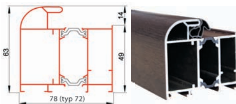
Ciepła ościeżnica aluminiowa z uszczelką do drzwi stalowych zewnętrznych 72 LUX, 72 LUX TERMO, 85 LUX TERMO PLUS
