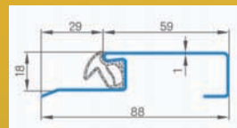
Próg z stali nierdzewnej z uszczelką
